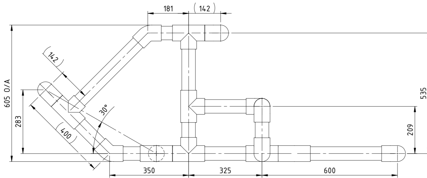
ELEVATION
